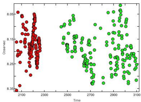
(3) HJD 2452056 - HJD 2452261 (red) HJD 2452447 - HJD 2453102 (green)
